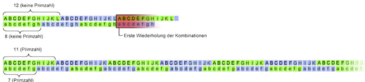
Abbildung 2: Dieses Schema verdeutlicht, wie Primzahlen im Wechsellnssystem unerwünschte Wiederholungen von Objektkombinationen vermeiden.
